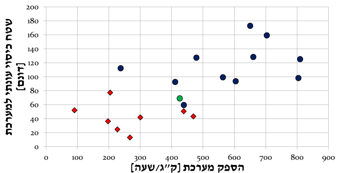
איור 7: שטח כיסוי עונתי למערכות גדודי ירוק ומכני.
