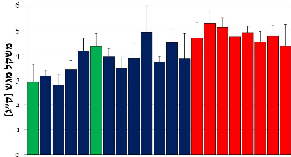
איור 3: משקל ממוצע למגש בגדיד ידני (אדום) מכני (כחול) ושרוולים (ירוק)
