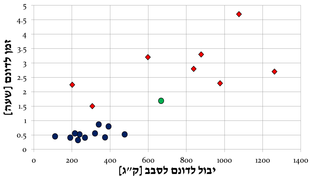
איור 4: השפעת היבול ומערכת הגדיד על הספק עבודה
