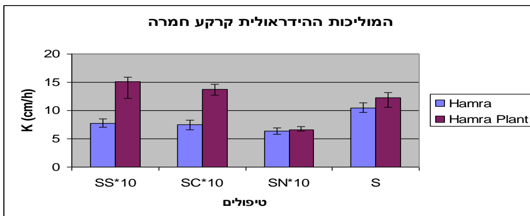
איור 15. השפעת הוספת הבוצות בשיעור של 500 ק"ג/ד' של חנקן על המוליכות ההידראולית ברוויה בשכבת הקרקע העליונה בעציצים. S – קרקע ביקורת בעציצים, SN – בוצה מיוצבת בסיד, SC – קומפוסט בוצה, SS – בוצה "דרג ב" מרעננה.
