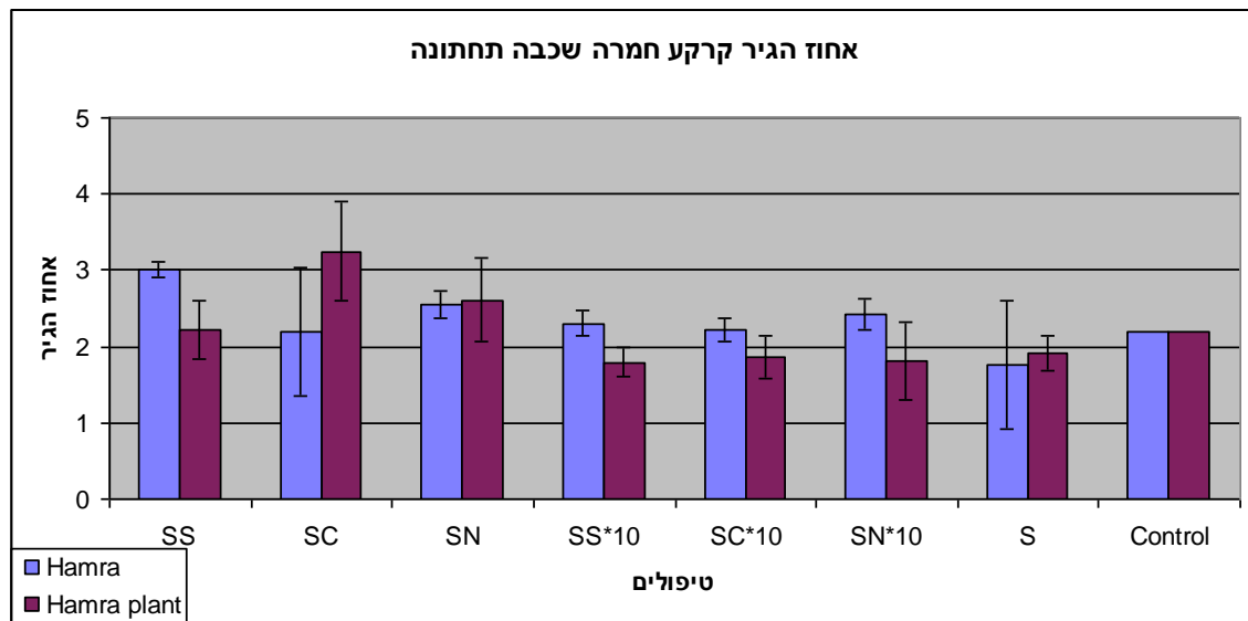
איור 3. השפעת הוספת הבוצות בשיעור של 50 ו-500 ק"ג/ד' של חנקן (10*) ונוכחות צמח על תכולת הגיר בשכבת הקרקע העליונה והתחתונה בקרקע חול-סייני. Control – קרקע מקורית, S – קרקע ביקורת בעציצים, SN – בוצה מיוצבת בסיד, SC – קומפוסט בוצה, SS – בוצה "דרג ב" מרעננה.
