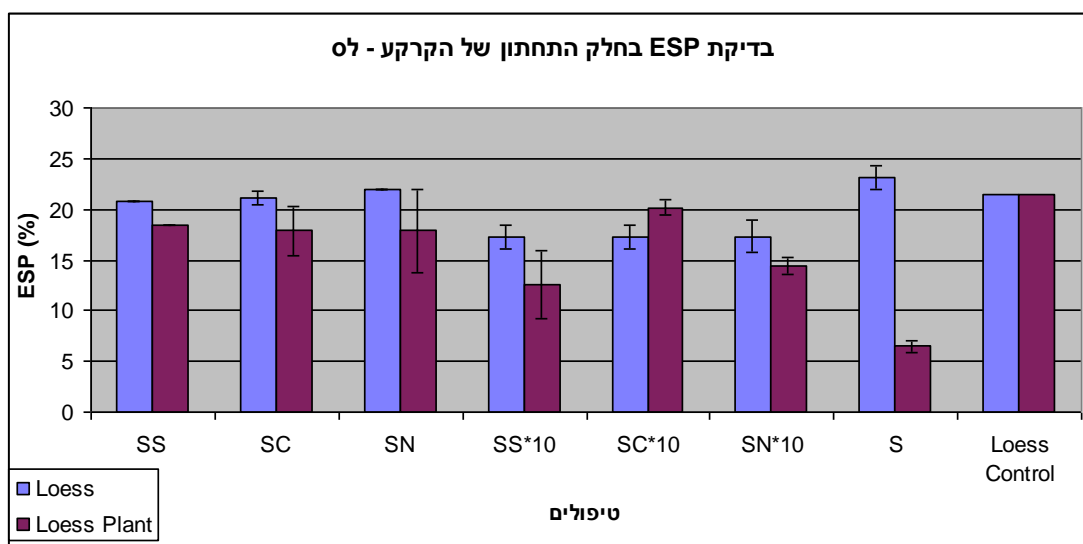
איור 8. השפעת הוספת הבוצות בשיעור של 50 ו-500 ק"ג/ד' של חנקן ( 10^* ) ונוכחות צמח על אחוז נתרן חליף (ESP) בשכבת הקרקע העליונה והתחתונה בקרקע טיין. Control – קרקע מקורית, S – קרקע ביקורת בעציצים, SN – בוצה מיוצבת בטיד, SC – קומפוסט בוצה, SS – בוצה "דרג ב" מרעננה.
