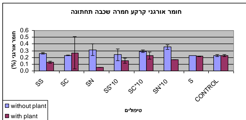
איור 6. השפעת הוספת הבוצות בשיעור של 50 ו-500 ק"ג/ד' של חנקן ( 10^* ) ונוכחות צמח על תכולת חומר אורגני בשכבת הקרקע העליונה והתחתונה בקרקע חול-סייני. Control – קרקע מקורית, S – קרקע ביקורת בעציצים, SN – בוצה מיוצבת בסיז, SC – קומפוסט בוצה, SS – בוצה "דרג ב" מרעננה.
