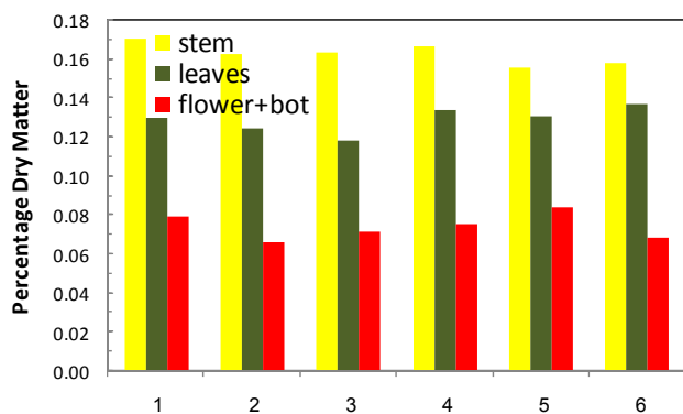
איור 11. משקל הצמח הכולל ומשקלי הגבעול, העלים והפרחים+חנטים (מימין) ופרקציית החומר היבש של הגבעול, העלים והפרחים+חנטי הגבעול, העלים והפרחים+חנטים (משמאל) ב-4 באוגוסט (למעלה) וב-4 בנובמבר (למטה) בששה הטיפולים של הניסוי
