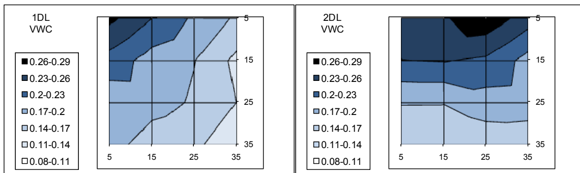
איור 1. פירוסי תכולת הרטיבות הנפחית (מדידות TDR) בניסוי חידור תמידי משלוחה בודדת (משמאל, מקור קווי של 107 סמ"ר/שעה) ומצמד שלוחות במרחק של 40 ס"מ ביניהן (מימין, מדידות רק בשלוחה הימנית) ללא צמחים (4 בדצמבר 2008). ממוצע של 3 חזרות.
