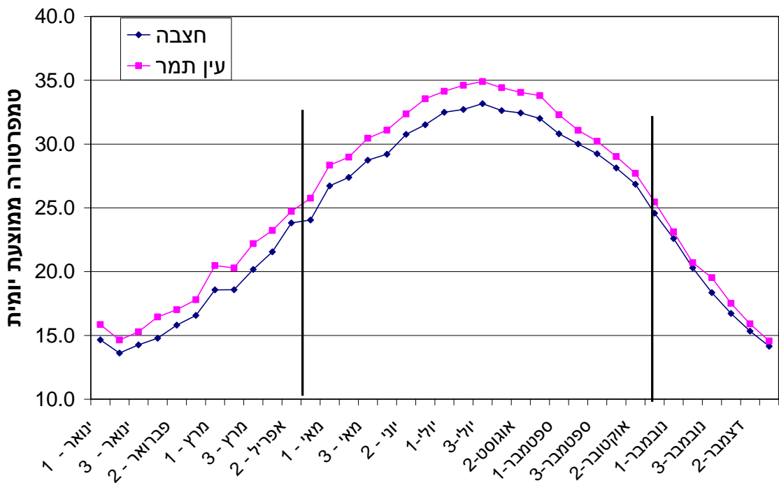
איור 3: ממוצע לשנים 1997-2007 של נתוני עשרת לטמפרטורת יום ממוצעת בחצבה ובעין תמר. הקווים האנכיים מסמנים את התחום שמתאים להערכתנו להתפתחות הקימחון בשדה, בטמפרטורות גבוהות התפתחות הפטרייה מעוכבת.
