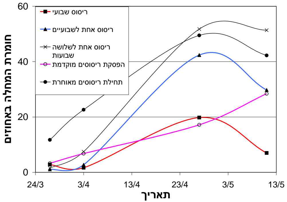
איור 2: התפתחות הקימחון על החלק התחתון של העלווה בטיפולי ריסוס שונים בהליוגופרית בניסוי אביב 2006.
