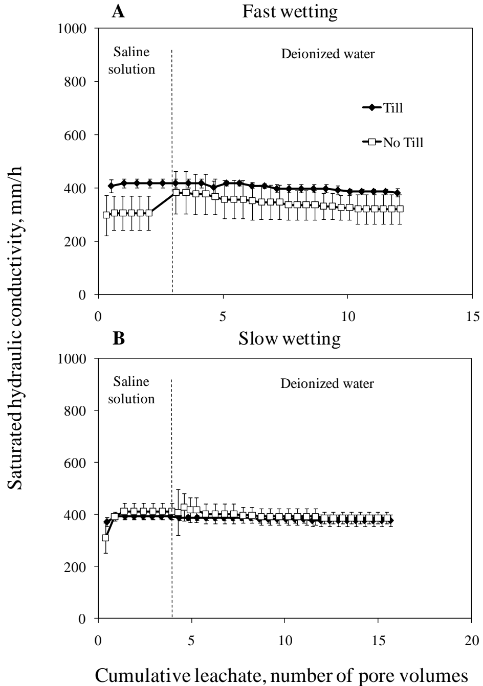
איור 2: ערכי מוליכות הידראולית ברוויה של קרקע חולית מבית דגן לאחר עיבוד בפליחה או באי-פליחה כתלות בנפח התשטיפ בשטיפה עם תמיסת מלח (Saline solution) ומים מזוקקים (Deionized water) בהרטבה מהירה (A) ואיטית (B). הקווים האנכים בגרפים הם ערכי סטיית התקן.
