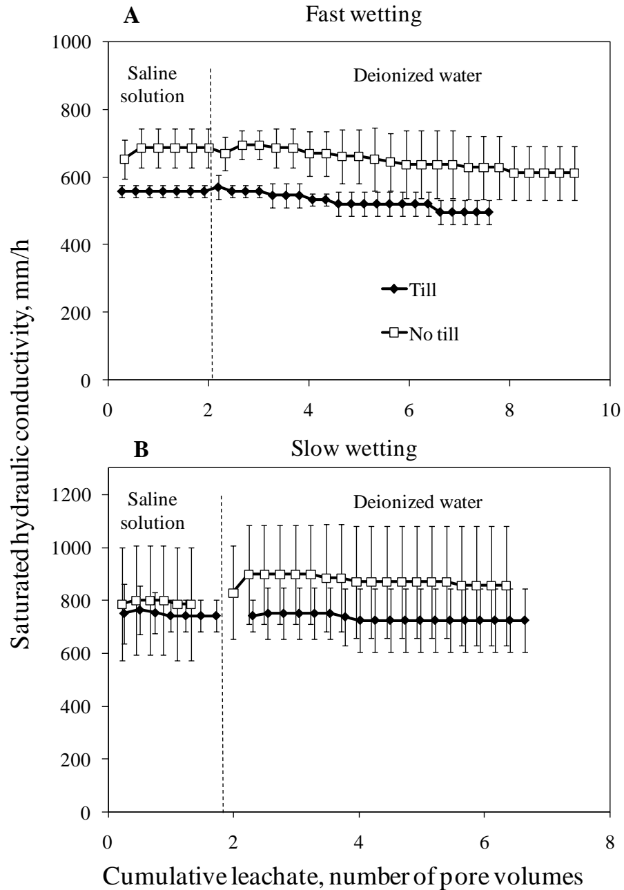
איור 1: ערכי מוליכות הידראולית ברוויה של קרקע חרסיתית מלביא לאחר עיבוד בפליחה או באי-פליחה כתלות בנפח התשטיפ בשטיפה עם תמיסת מלח (Saline solution) ומים מזוקקים (Deionized water) בהרטבה מהירה (A) ואיטית (B). הקווים האנכים בגרפים הם ערכי סטיית התקן.
